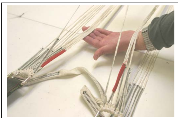
Abb. 6 Leinenkontrolle
